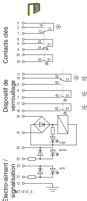
Fig. 1 : Gâche à l'état désactivé: - YRXKM: électro-aimant verrouillé, actionneur retirée, porte ouverte - YRXK01M: électro-aimant verrouillé, actionneur retirée, clé insérée, porte ouverte
