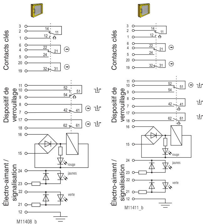
Fig. 1 : Gâche à l'état désactivé: - YRXKM: électro-aimant verrouillé, actionneur retirée, porte ouverte - YRXK01M: électro-aimant verrouillé, actionneur retirée, clé insérée, porte ouverte
