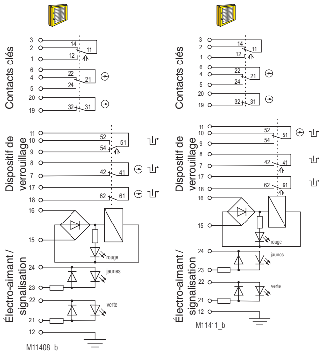
Fig. 1 : Gâche à l'état activé: électro-aimant verrouillé, clé insérée
