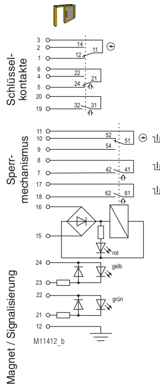
Bild 1: Zuhaltung im aktivierten Zustand: Magnet verriegelt, Schlüssel gesteckt
