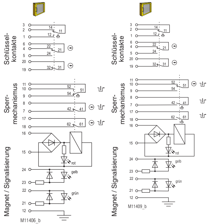
Bild 1: Zuhaltung im aktivierten Zustand: Magnet verriegelt, Schlüssel gesteckt
