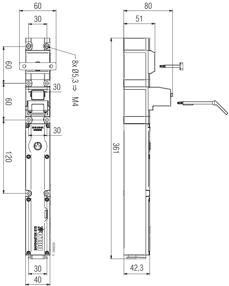
ZRH01BM/K Tolérances générales ± 2%
