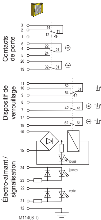
Fig. 1 : Verrouillage à l'état activé: électro-aimant verrouillé, actionneur et clé insérés
