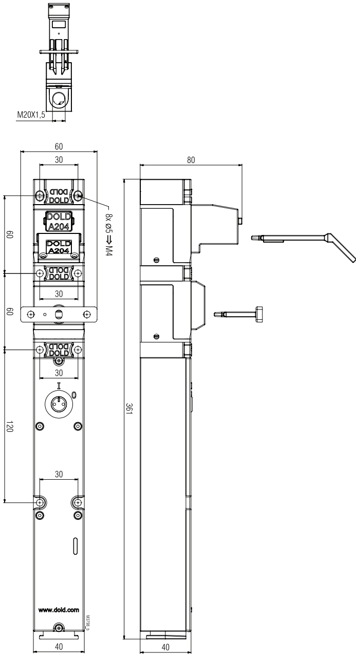
ZRHB01M/K Tolérances générales ± 2%
