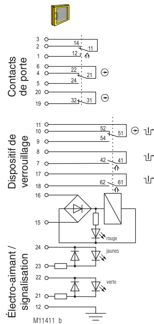
Fig. 2 : Verrouillage à l'état désactivé: Électro-aimant déverrouillé, actionneur et clé insérés
