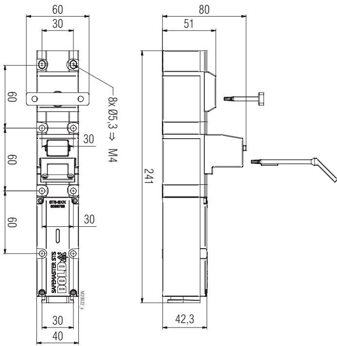
SX01BM/K Tolérances générales ± 2%
