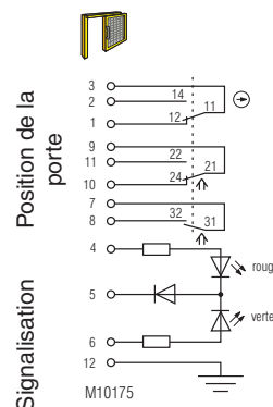
Fig. 2 : Verrouillage à l'état désactivé: clé retirée porte ouverte
